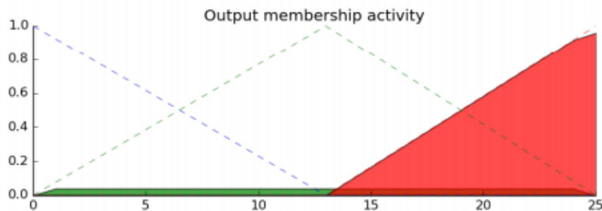
Gambar 2.3 Output membership activity yang harus dikombinasikan ( aggregation )
