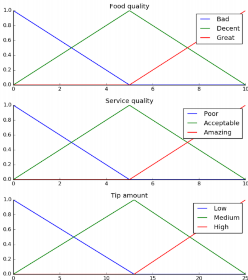
Gambar 2.2 Desain fuzzy logic untuk membership function untuk pemberian tip.
